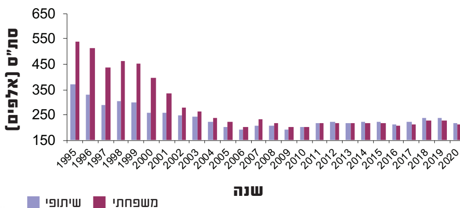
ממוצע סת"ס ארצי לפי נתוני שיווק חלב, לפי שנים ומגדר
