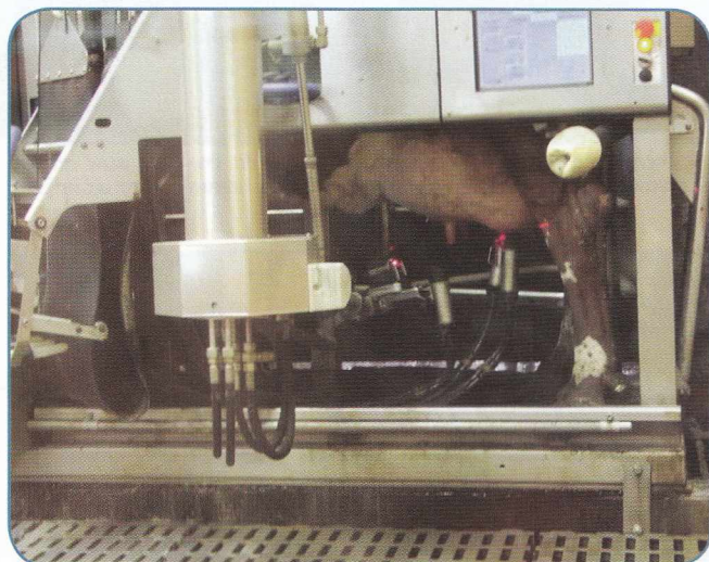
מערכת החליבה האוטומטית - רובוט החליבה השוודי
