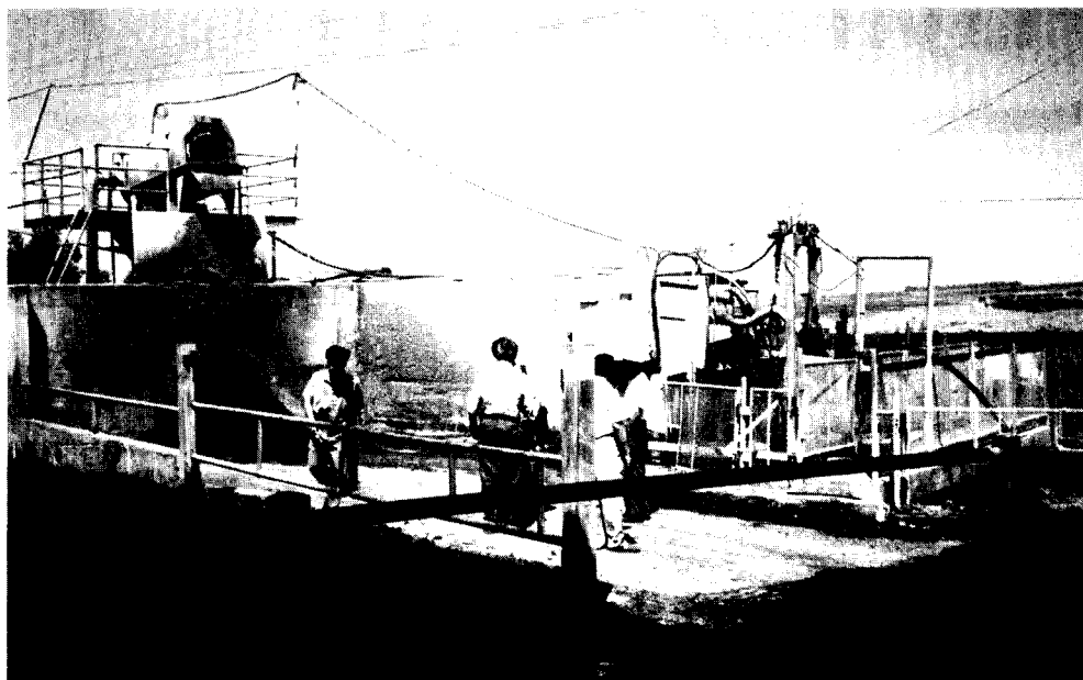
המתקן להפרדת זבל ברפת עין חרוד איחוד.
