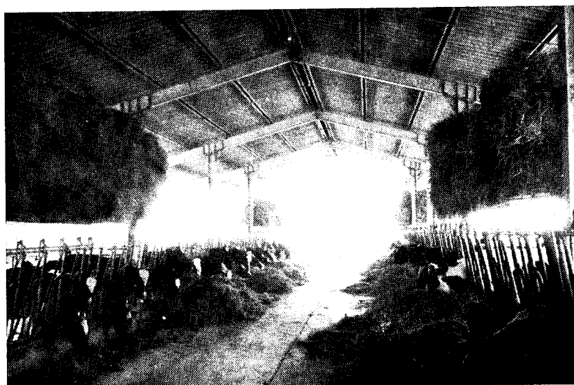
סככה להחזקת בקר כמקובל ברפתות מודרניות באיטליה.
