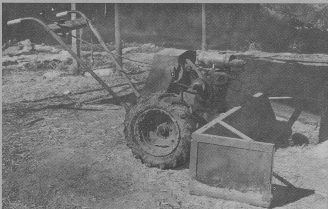
מיתקן-יד ממונע לניקוי משטחי ביטון מזבל במשק מרכס במושב אורות (צילם : אלי סמסון)
