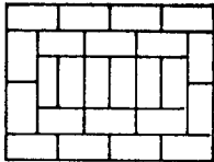
תנוחת השכבות — 6, 3
