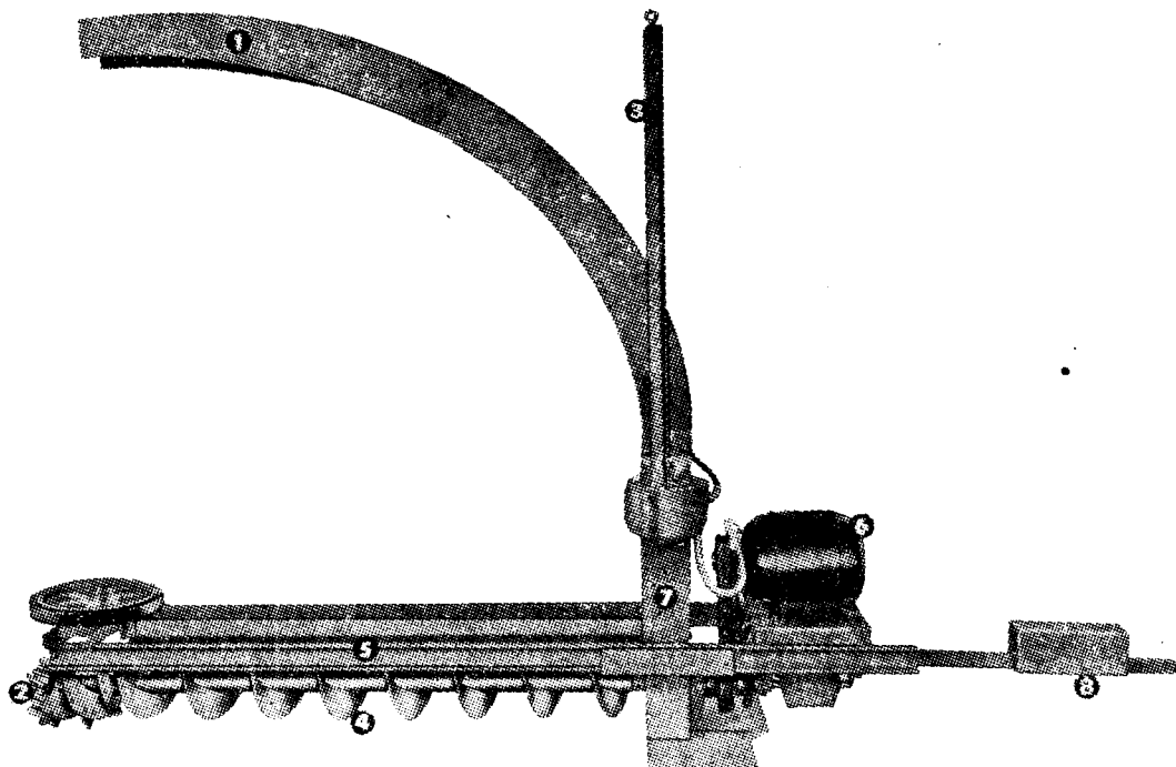
פורק התחמיץ שהותקן בעין המפרץ 1. מרזב ספיקה; 2. מנקה הקירות; 3. ייצול; 4. חלזון 9"; 5. מסגרת 80 מ"מ; 6. מנוע חשמלי; 7. שרוול; 8. משקולת נגדית; 9. גלגל הנעה; 10. גלגלי הולכה.
