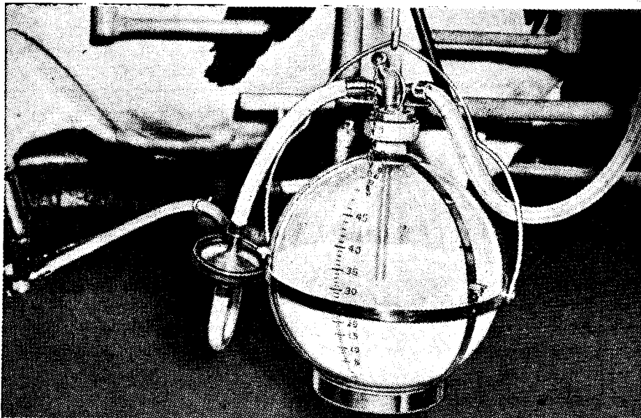
צנצנת Chore Boy ללא ברז, בגמר החליבה הופכים אותה, והיא מתרוקנת מאליה. הרחיצה במקום.
