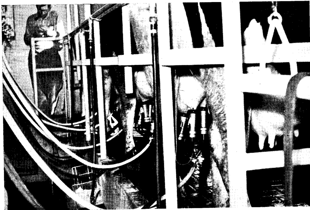
הופעל בית חליבה ראשון בארץ מטיפוס "שדרת-הדג" (ראה רשימה עמוד 9)
